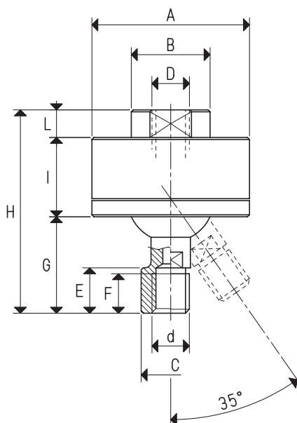
GIUNTI A SNODO POSIZIONABILI CON CONNESSIONE VUOTO ASSIALE
