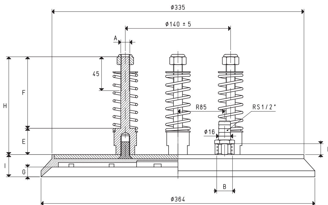
VENTOSA CON SUPPORTO VULCANIZZATO
